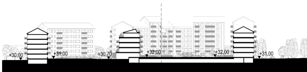
Bild 12 Sektion som visar den föreslagna bebyggelsen uppdelat i två kvarter. Här visas nya och anslutande markhöjder samt det delvis nedgrävda garaget. Bild Krook & Tjäder.
