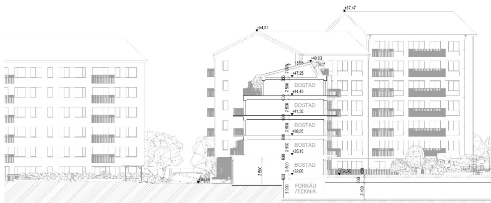
Bild 11. Sektion som visar den föreslagna lägre byggnaden med indraget våningsplan. Bild Krook & Tjäder.
