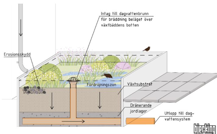
Bild 23. Illustration över hur en regnbädd fungerar. Bild: Bjerkning.
