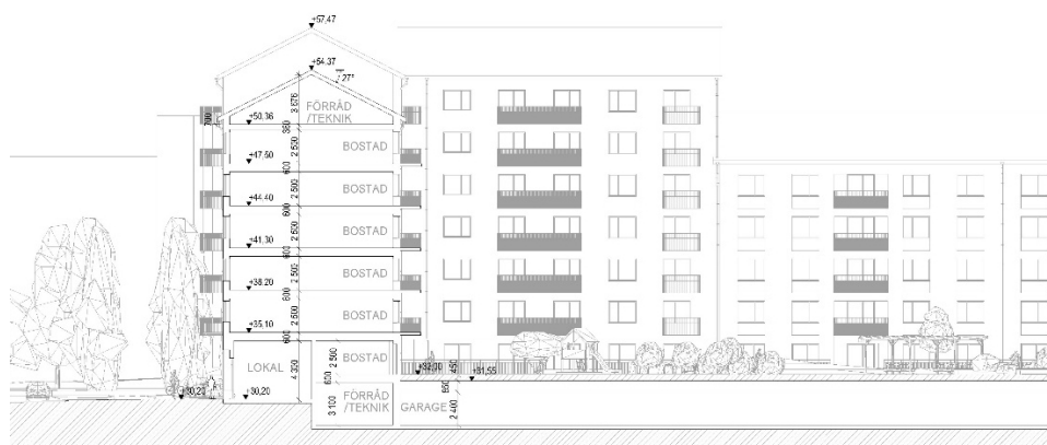
Bild 10. Illustration som visar sektioner för den nya föreslagna bebyggelsen med sex våningar med möjlighet för lokaler i bottenvåningen. Här visas en variation i höjd på föreslagen bebyggelsen. Bild Krook & Tjäder.
